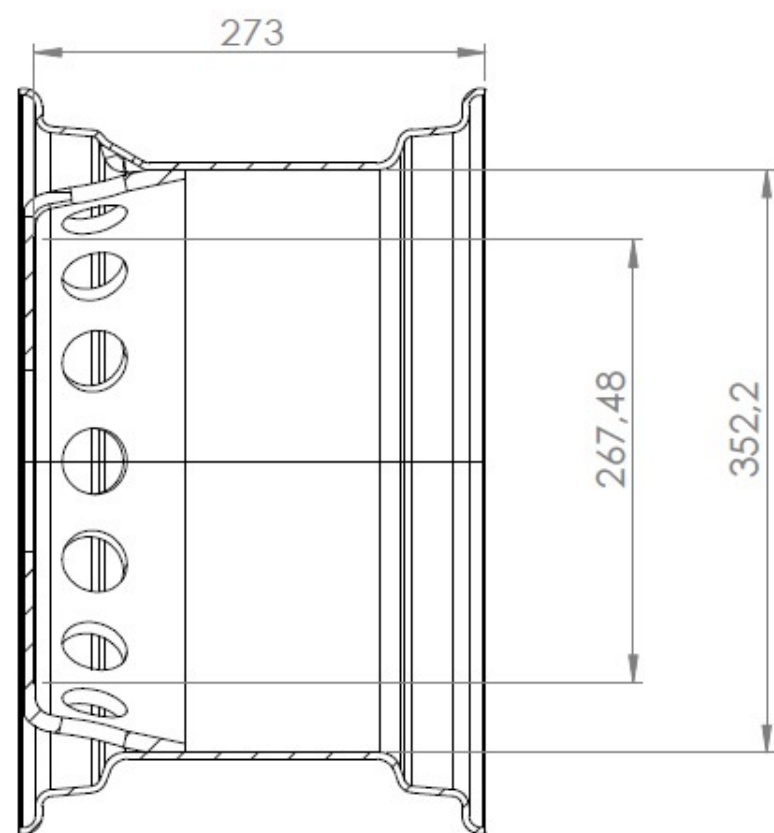
COUPE A-A
