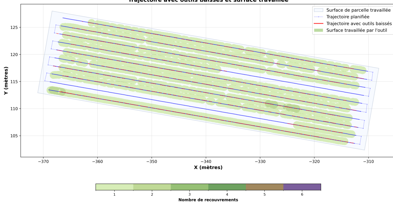
Trajectoire avec outils baissés et surface travaillée
