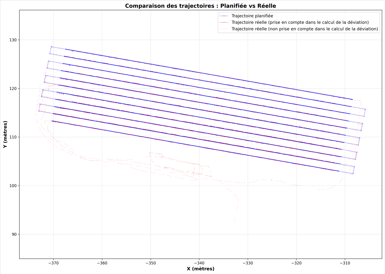
Figure 1.1: Comparaison trajectoire planifiée vs réelle
