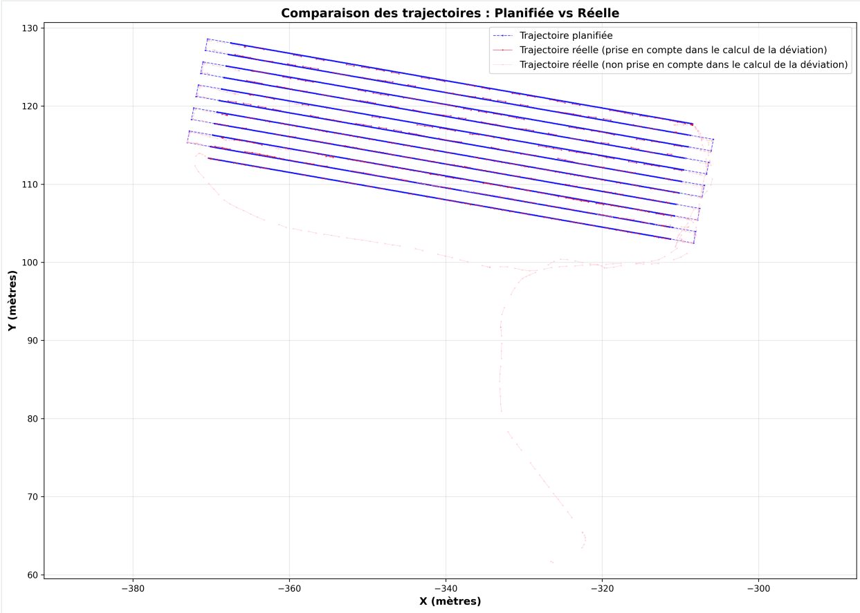
Figure 3.1: Comparaison trajectoire planifiée vs réelle
