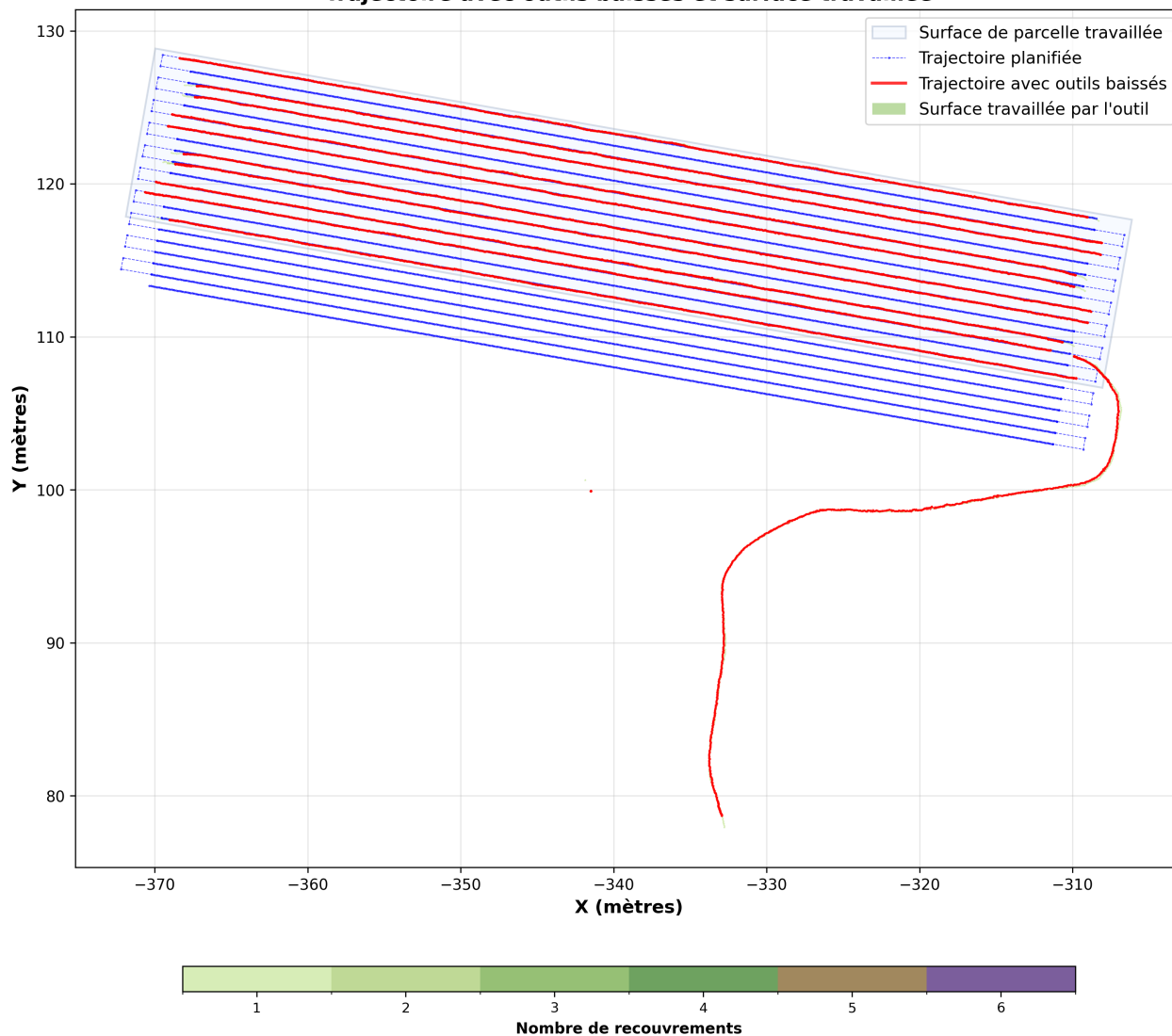
Trajectoire avec outils baissés et surface travaillée
