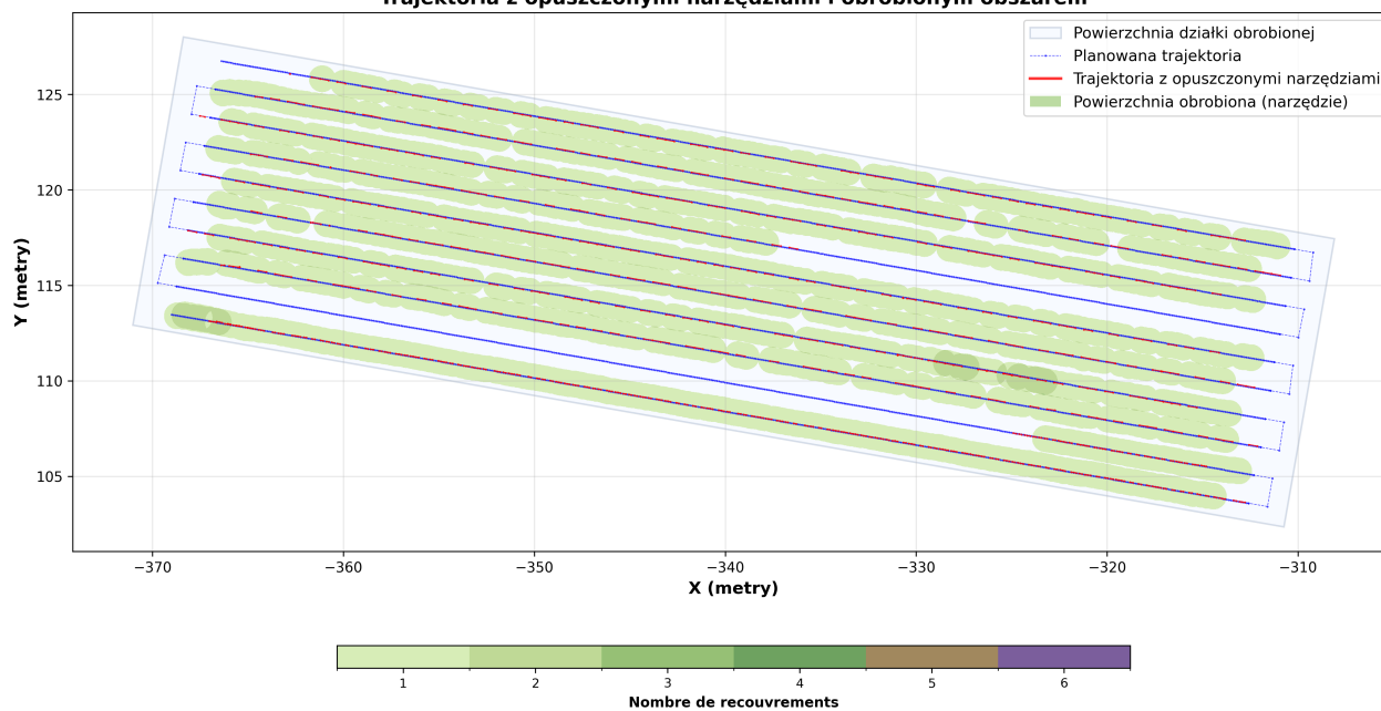
Trajektoria z opuszczonymi narzędziami i obrobionym obszarem
