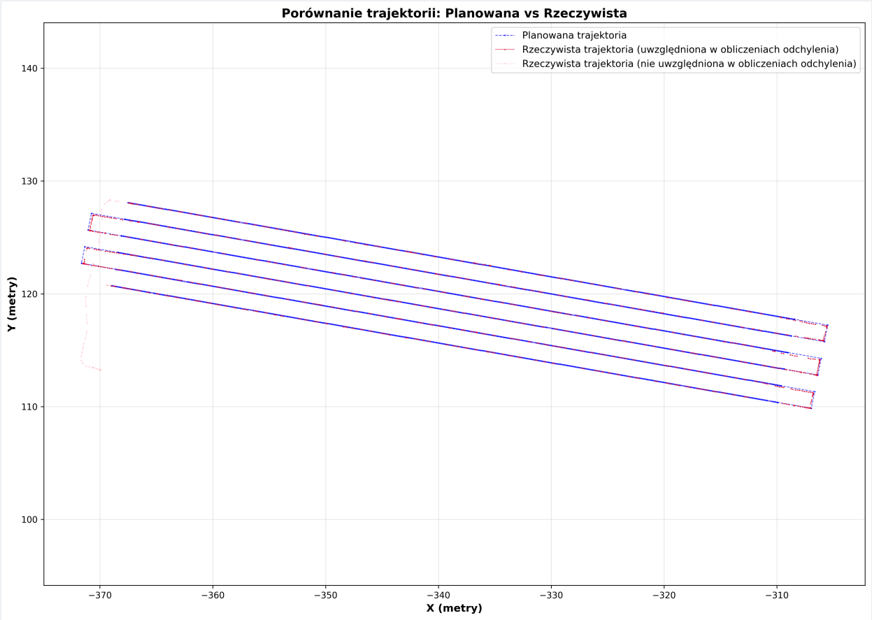
Wykres 2.1: Porównanie planowanej vs rzeczywistej trajektorii
