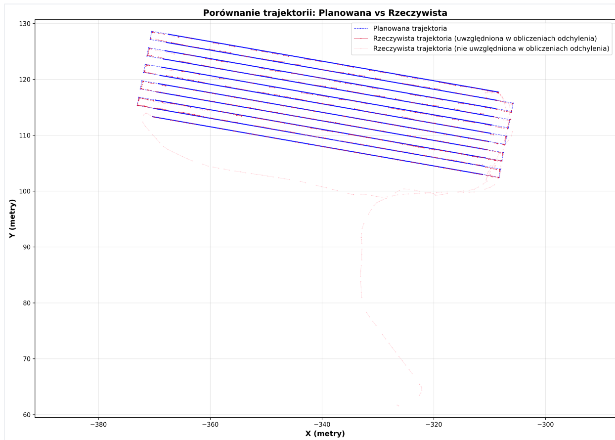
Wykres 3.1: Porównanie planowanej vs rzeczywistej trajektorii
