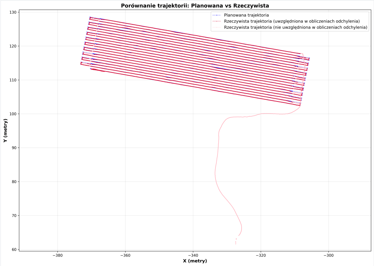
Wykres 4.1: Porównanie planowanej vs rzeczywistej trajektorii
