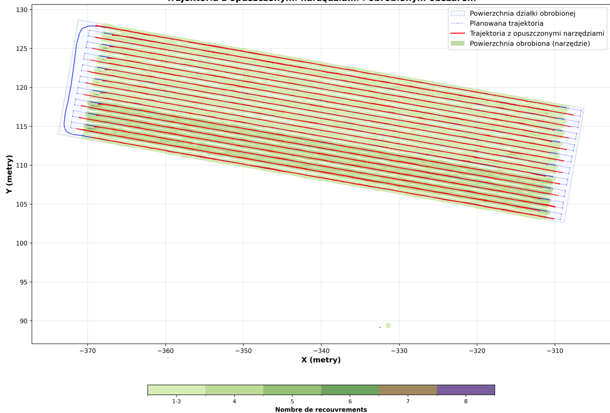
Trajektoria z opuszczonymi narzędziami i obrobionym obszarem
