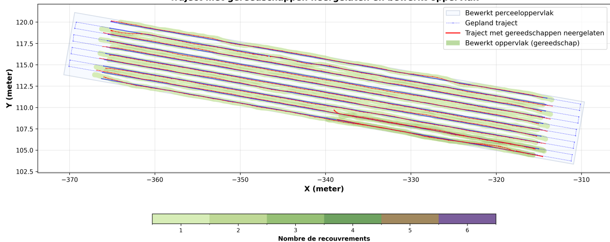
Traject met gereedschappen neergelaten en bewerkt oppervlak
