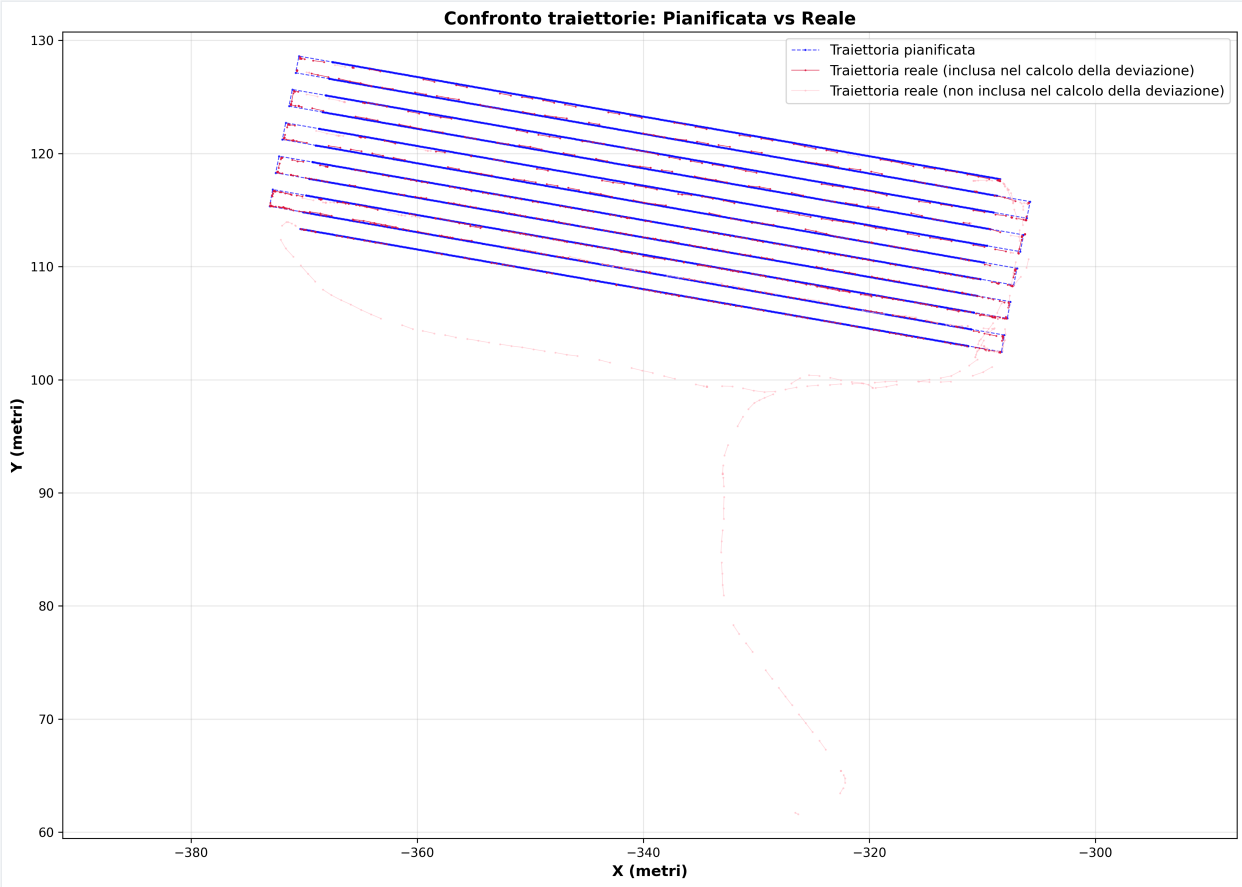
Figura 3.1: Confronto traiettoria pianificata vs reale
