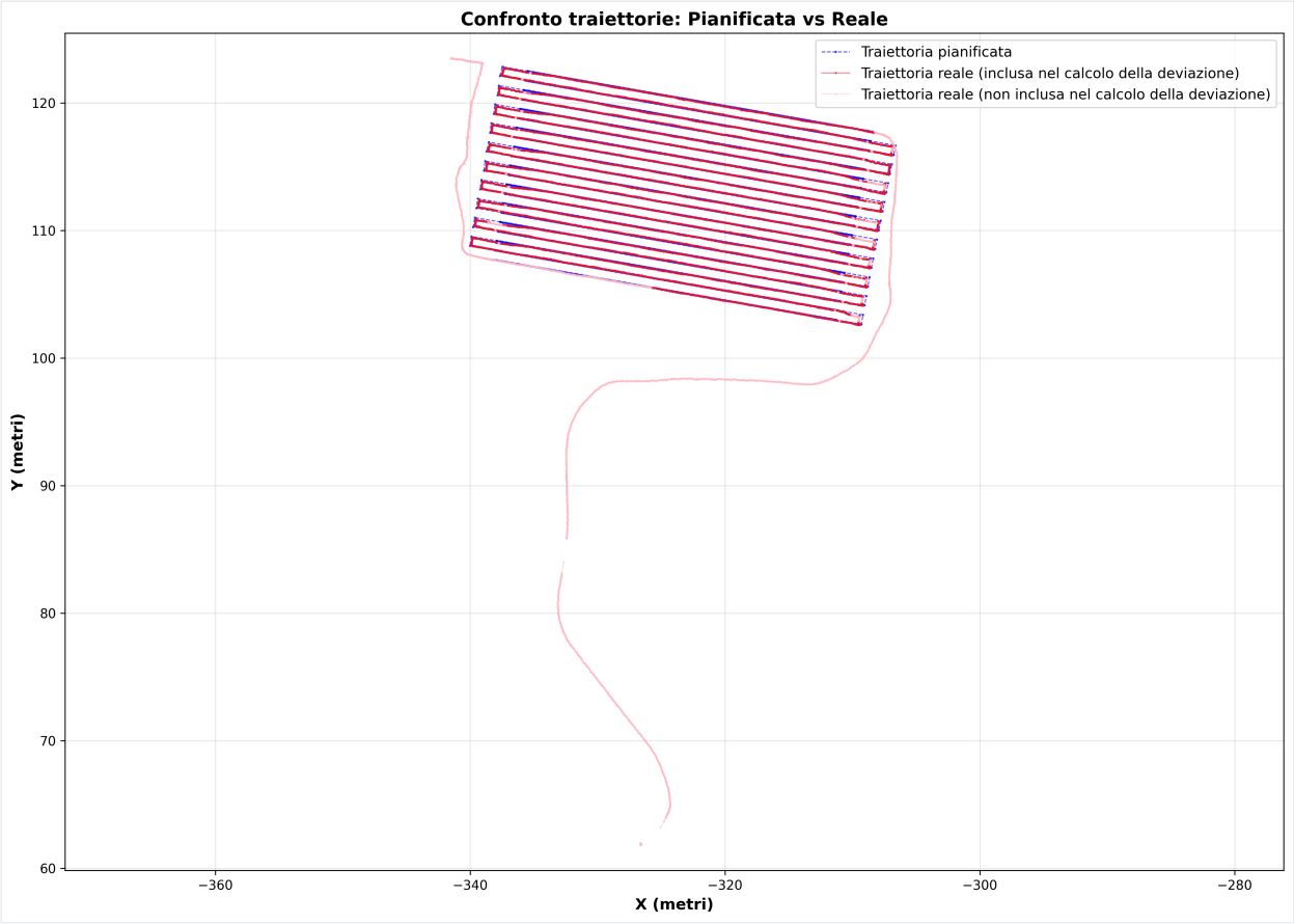
Figura 2.1: Confronto traiettorie pianificate vs reale
