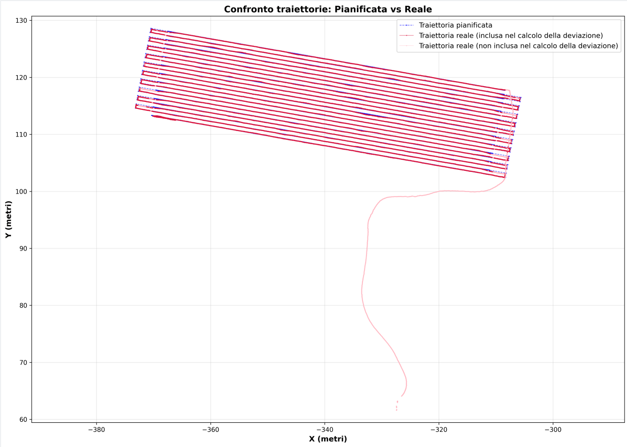
Figura 4.1: Confronto traiettoria pianificata vs reale
