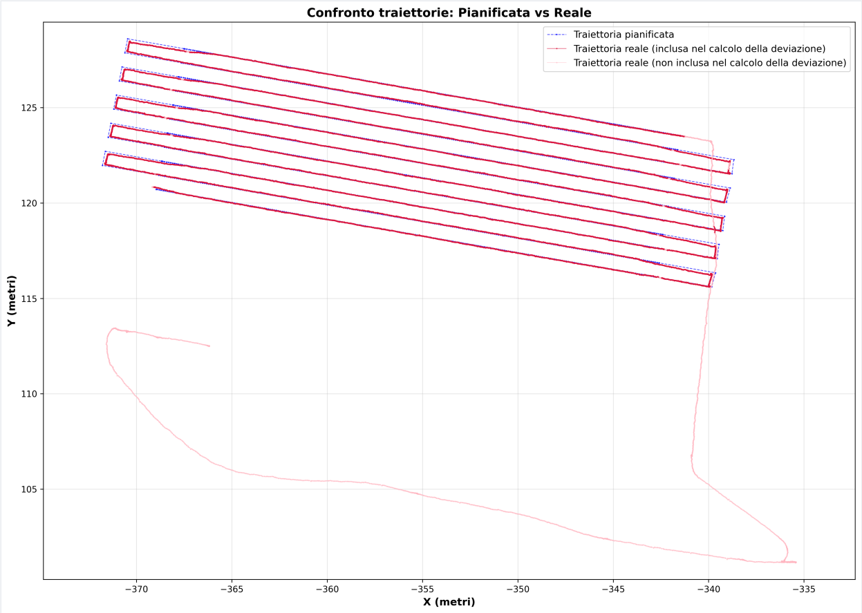
Figura 3.1: Confronto traiettoria pianificata vs reale
