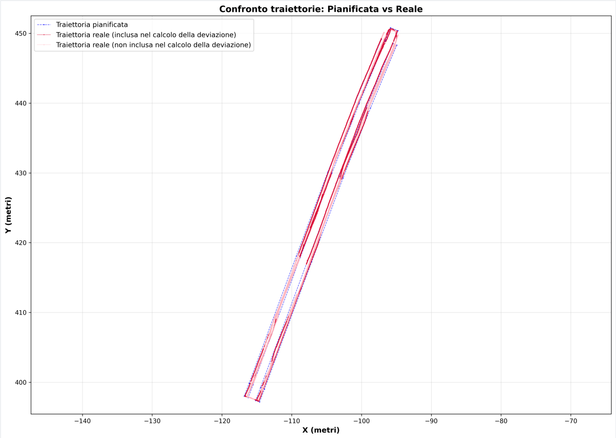
Figura 2.1: Confronto traiettoria pianificata vs reale
