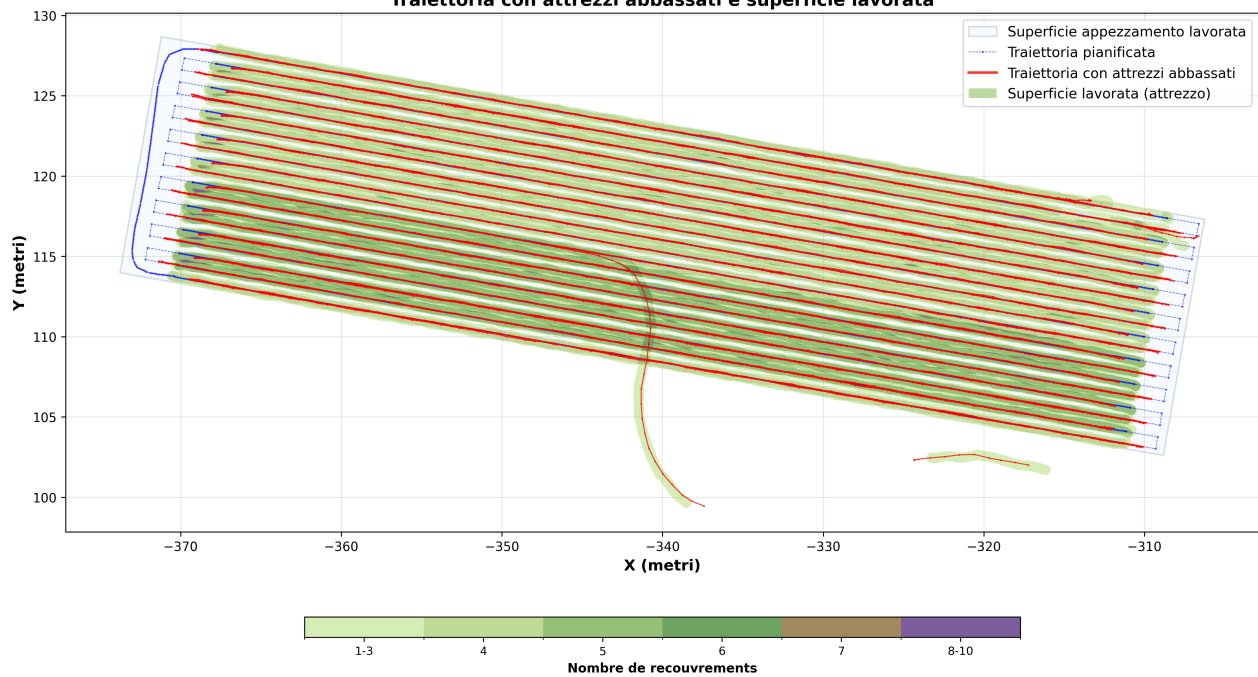
Traiettoria con attrezzi abbassati e superficie lavorata
