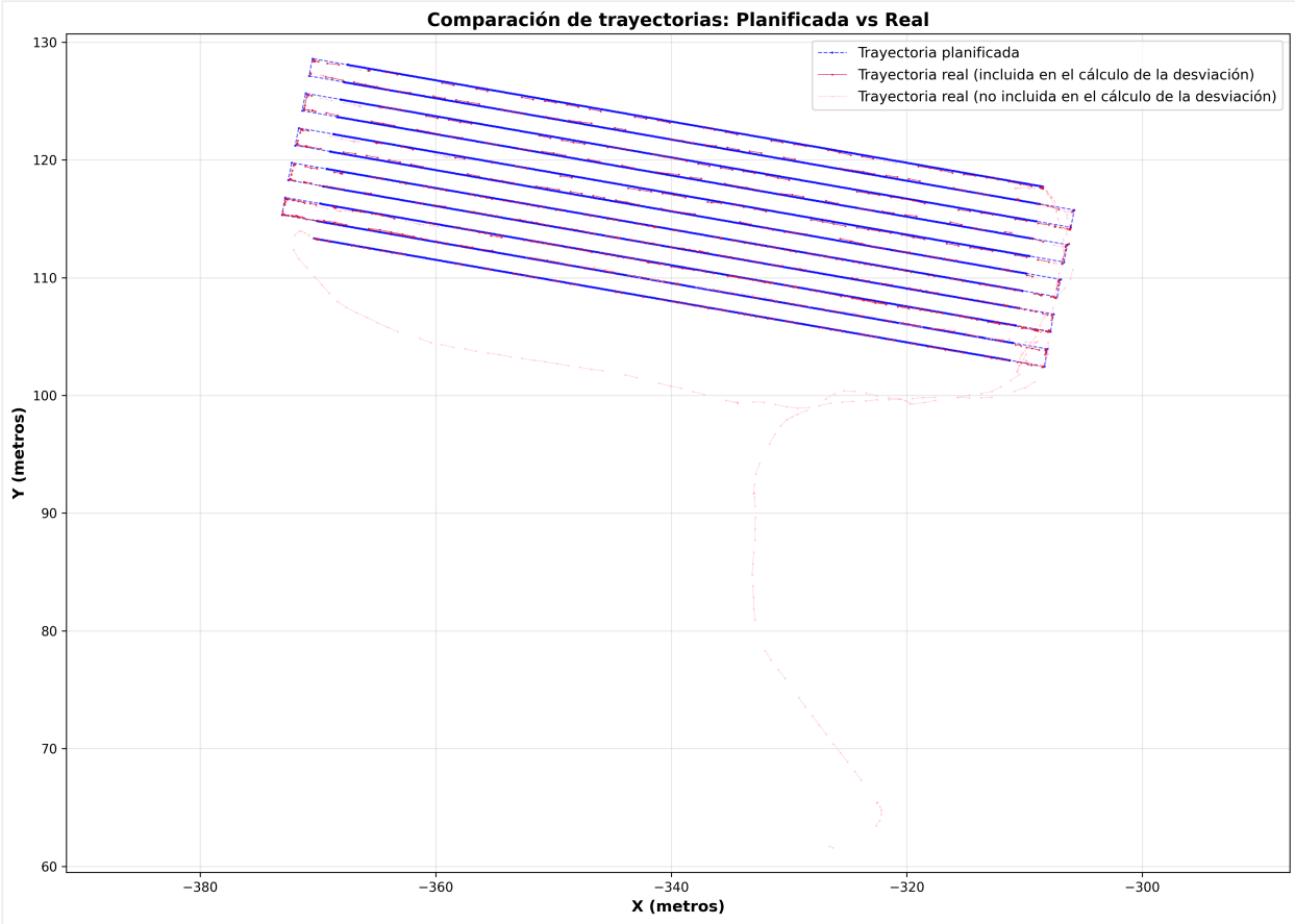
Figura 3.1: Comparación de la trayectoria planificada versus real
