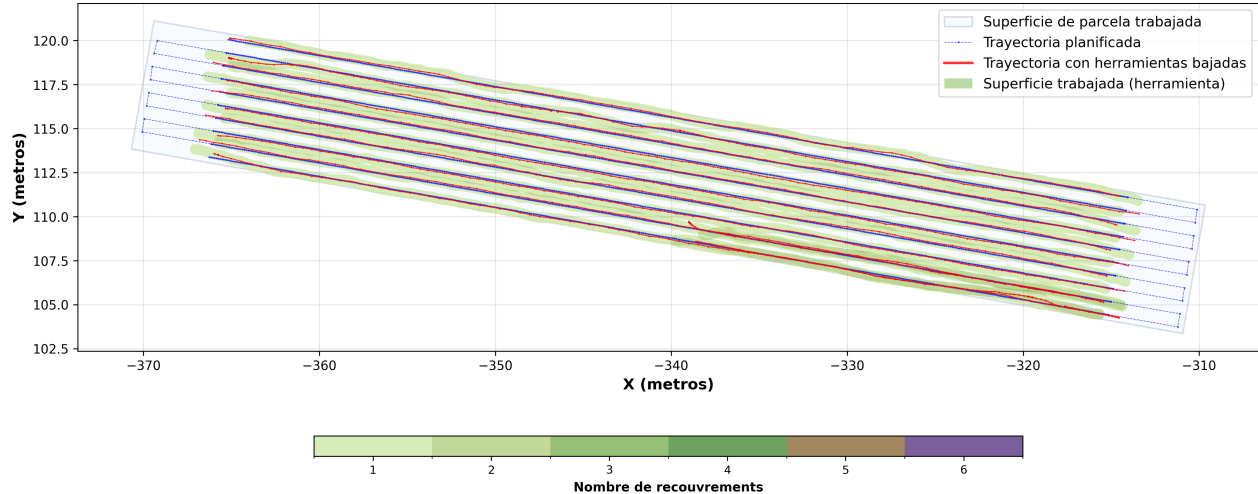
Trayectoria con herramientas bajadas y superficie trabajada
