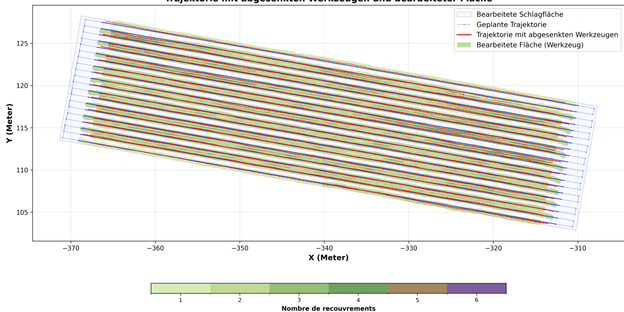
Trajektorie mit abgesenkten Werkzeugen und bearbeiteter Fläche
