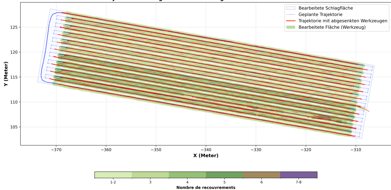
Trajektorie mit abgesenkten Werkzeugen und bearbeiteter Fläche
