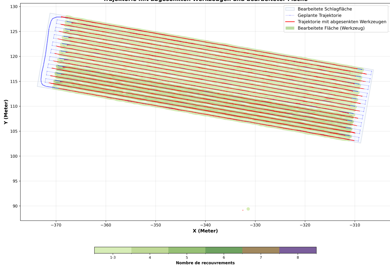
Trajektorie mit abgesenkten Werkzeugen und bearbeiteter Fläche
